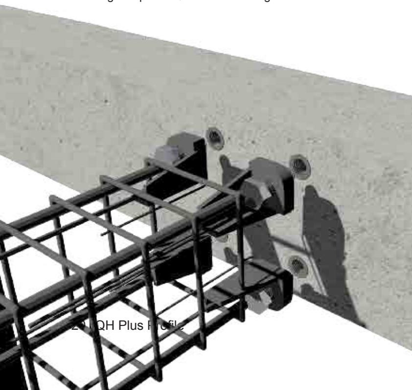
Kết nối cấu kiện bê tông dầm và dầm bằng sản phẩm QH Insert và Flange
